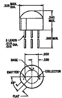
Q1 & Q2 EN2222 TO-105 PACKAGE
