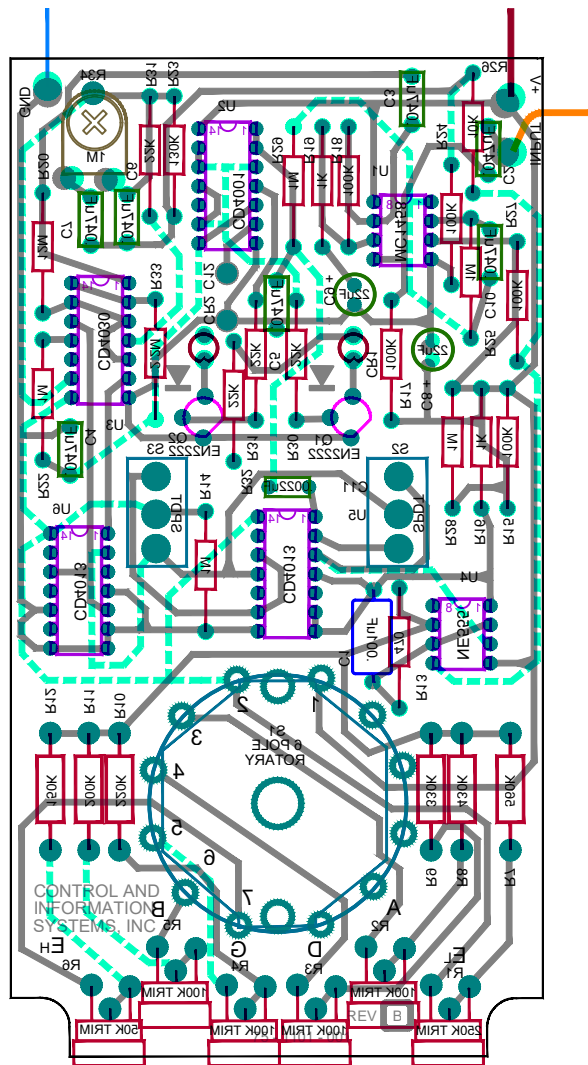
BOTTOM SIDE
