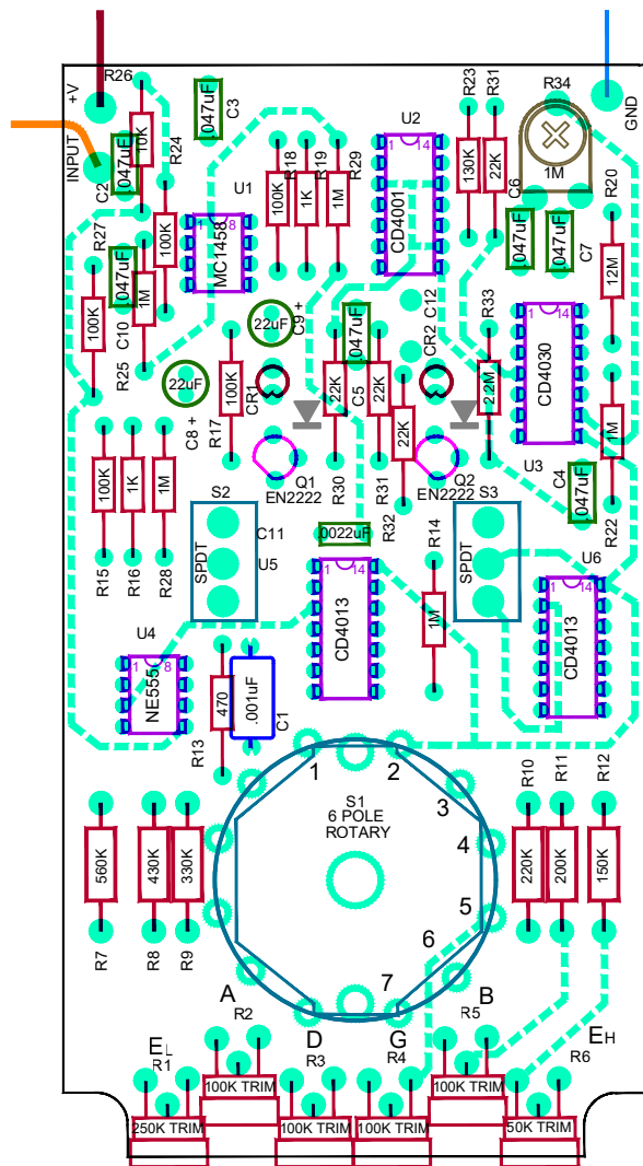
TOP SIDE
