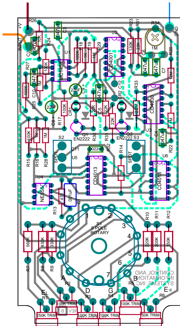
TOP SIDE
