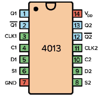
U5 & U6 CD4013 DUAL D FLIP-FLOP
