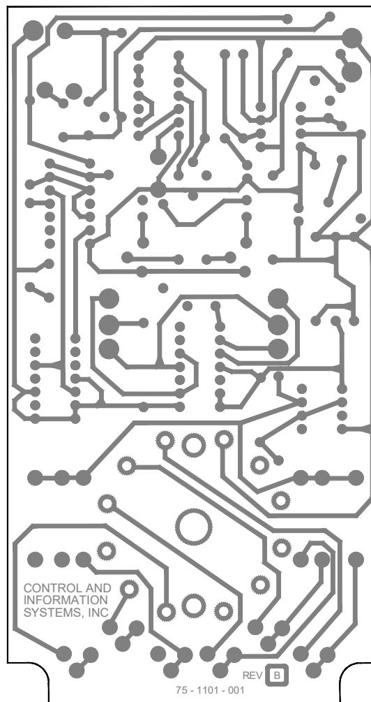
BOTTOM SIDE
